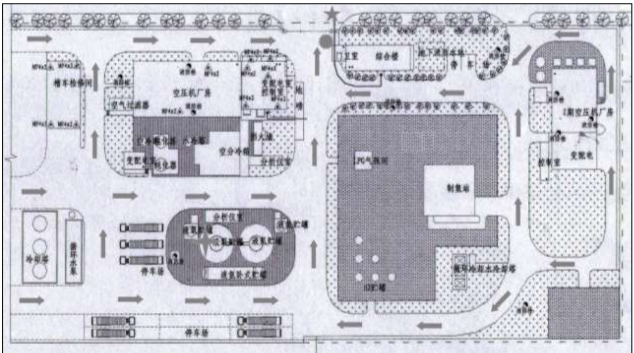
厂区紧急疏散路线图
